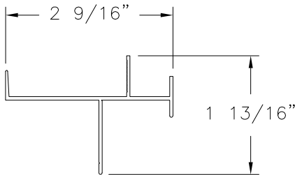
SILL (318-A) ALUMINUM 6063-T5
