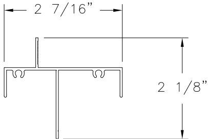
JAMB (319-A) ALUMINUM 6063-T5
