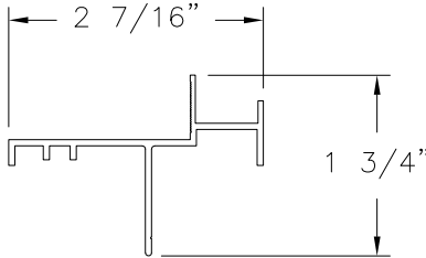
HEAD (320-A) ALUMINUM 6063-T5
